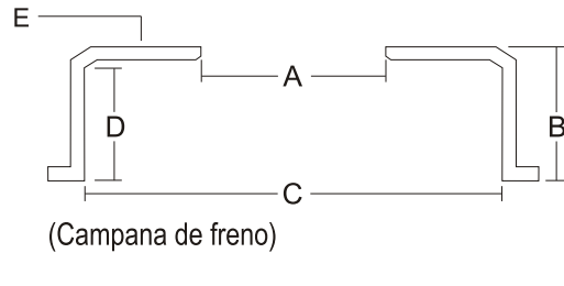
(Campana de freno)
